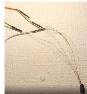
結線例
